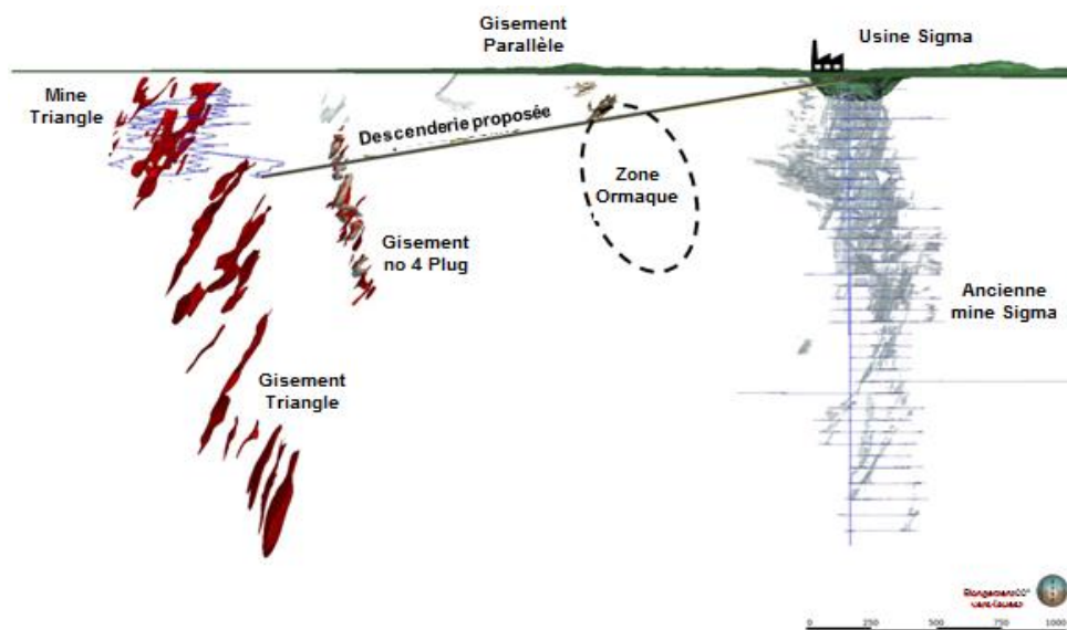
Figure 1 : Vue en coupe de la rampe proposée entre l'usine Sigma et la mine Triangle
