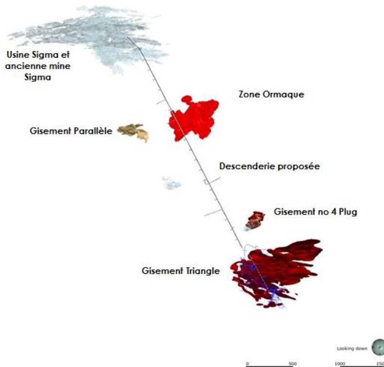
Figure 2 : Vue en plan de la rampe proposée entre l'usine Sigma et la mine Triangle
